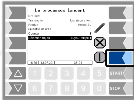
Commencer la livraison
